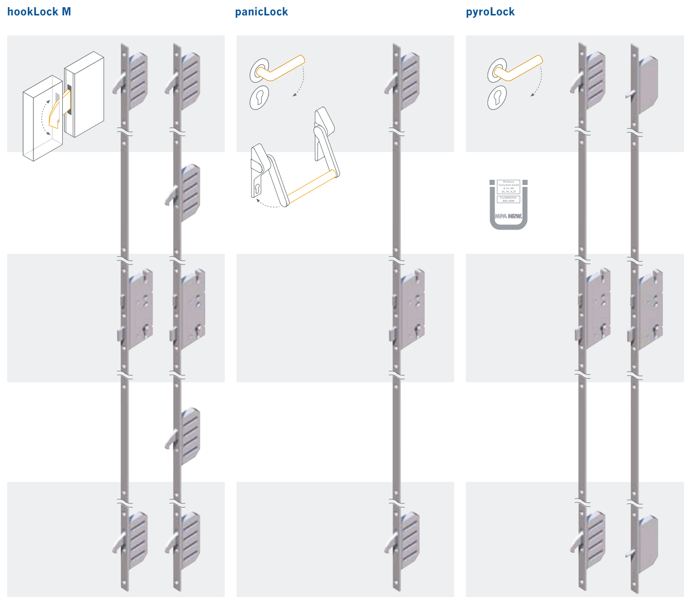
hookLock M – zamek z masywnymi ryglami
