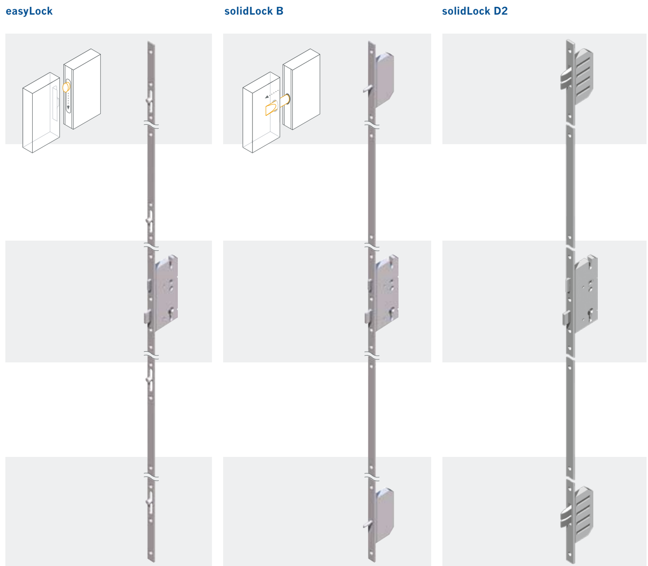
easyLock – zamek z rolkami lub trzpieniami grzybkowymi
